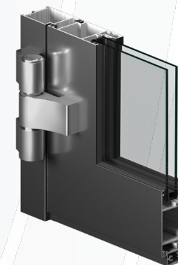
Ближний разрез нашего дверного профиля.
