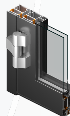
Ближний разрез нашего дверного профиля.
