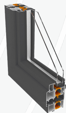
Ближний разрез нашего оконного профиля.
