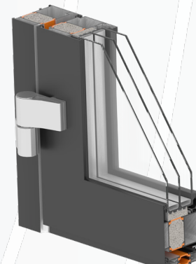
Ближний разрез нашего дверного профиля.
