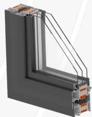
Ближний разрез нашего оконного профиля.
