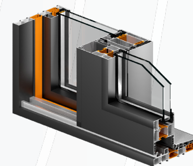
Задний вид нашей системы PSL (Pull and Slide).
