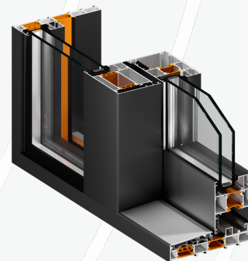
Передний вид нашей раздвижной системы PSL (Pull and Slide)
