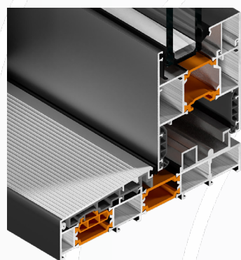
Ближний взгляд на разрез.
